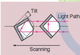
CCM 貓眼式稜鏡
